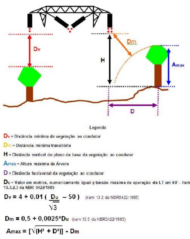
Figura 1.56. Fórmula para cálculo de distâncias copa x condutor.
