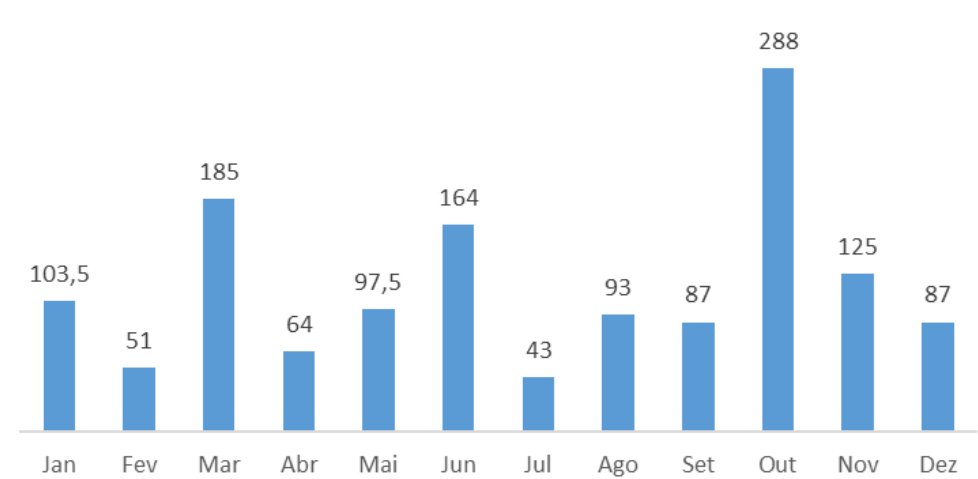
Figura 1.38. Registro mensal da precipitação pluviométrica em 2022.
