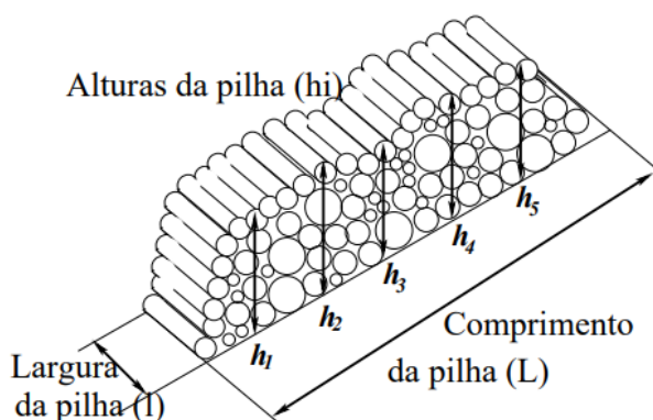
Figura 1.57. Representação da pilha de lenha e seus pontos de medição.
